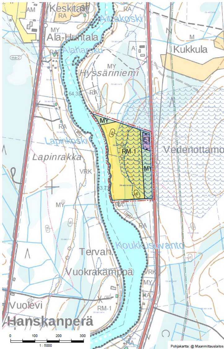
Kuva 12. Lapinkosken osayleiskaavaluonnos
